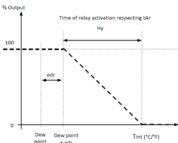
Figura 33: Punto di rugiada - Umidostato
