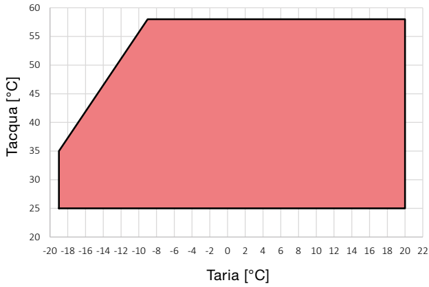
MODALITÀ RISCALDAMENTO HP_OWER 500RK - HP_OWER 500RK A400
