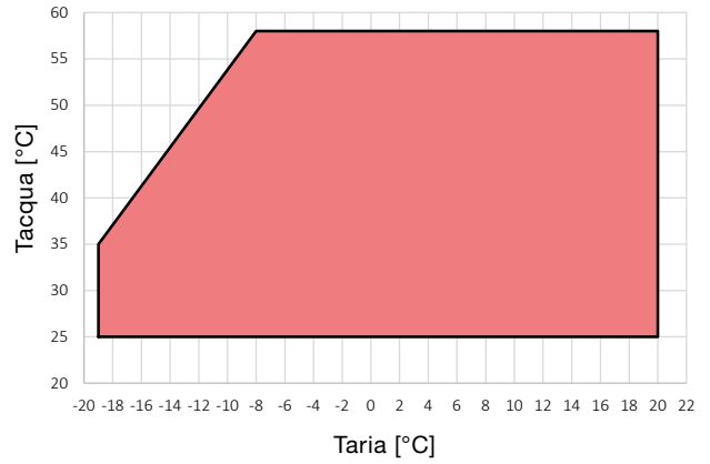
MODALITÀ RISCALDAMENTO HP_OWER 700RK - HP_OWER 700RK A400
