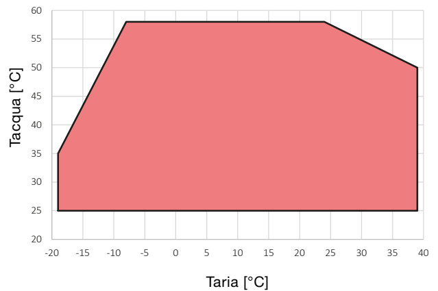
MODALITÀ SANITARIA HP_OWER 700RK - HP_OWER 700RK A400
