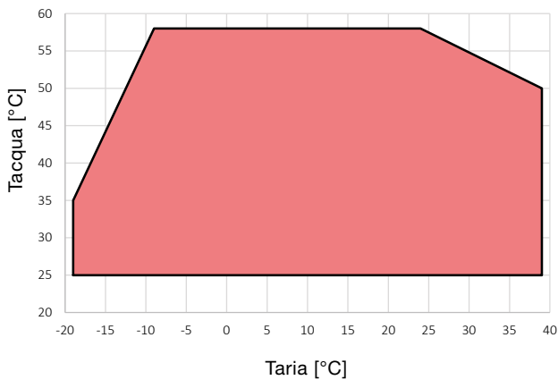
MODALITÀ SANITARIA HP_OWER 500RK - HP_OWER 500RK A400
