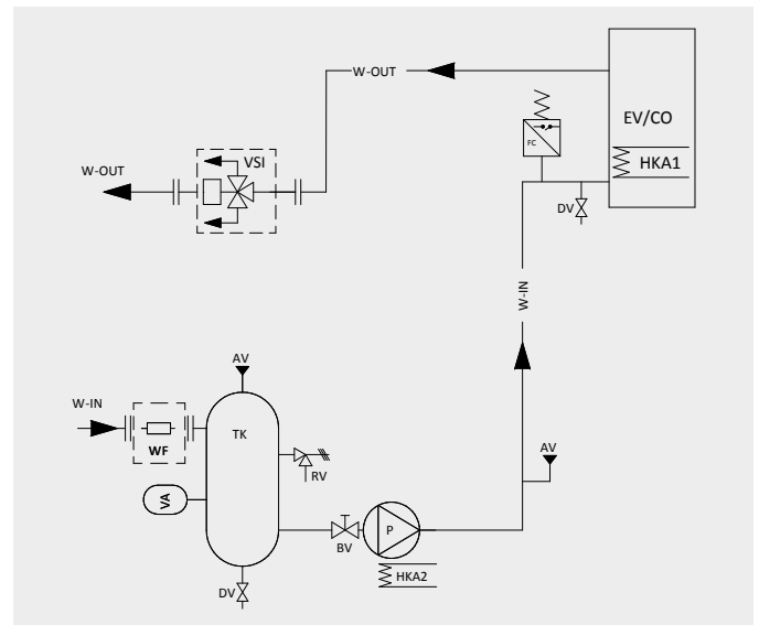
CIRCUITO IDRONICO VERSIONE A400
