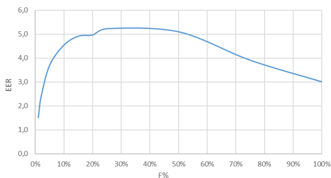
EER a carico parziale
